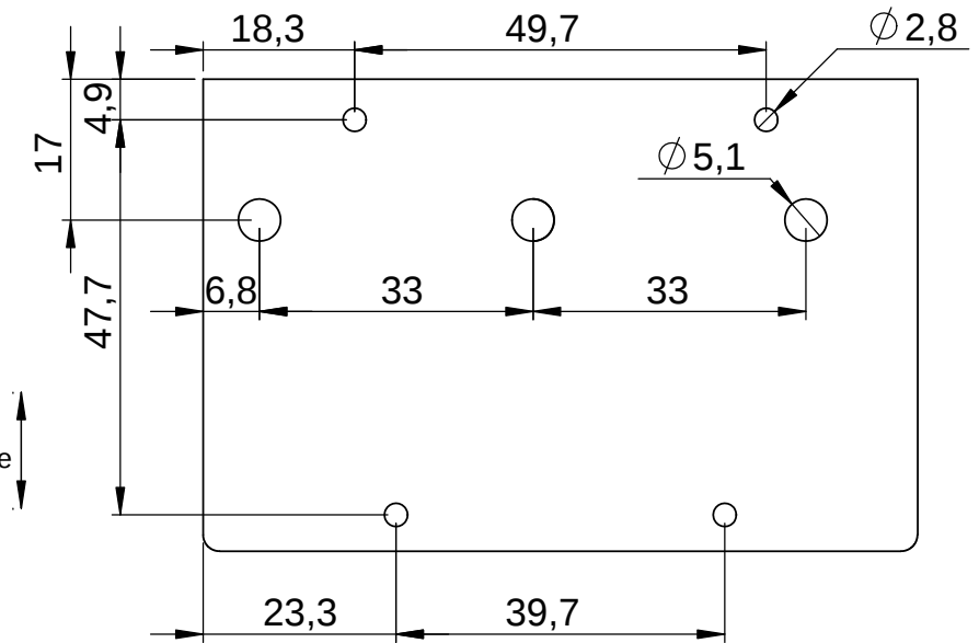
Untersicht bottom view
